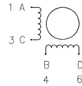
接线图 Wiring Diagram
